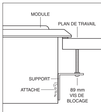
Supports d'installation
